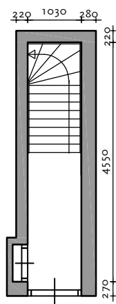
Begane grond
