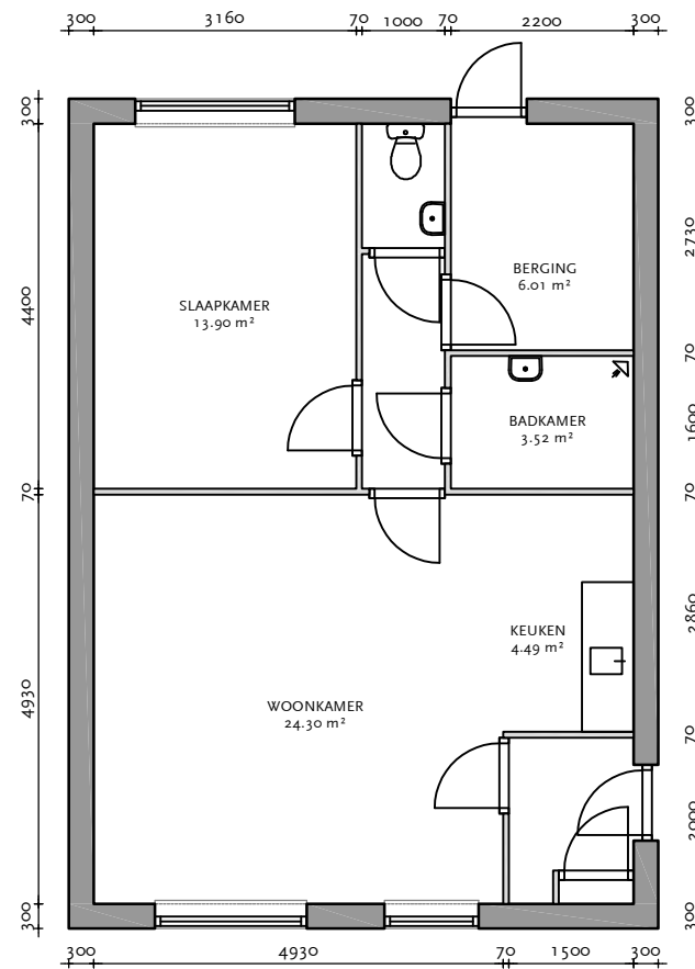
Begane grond
